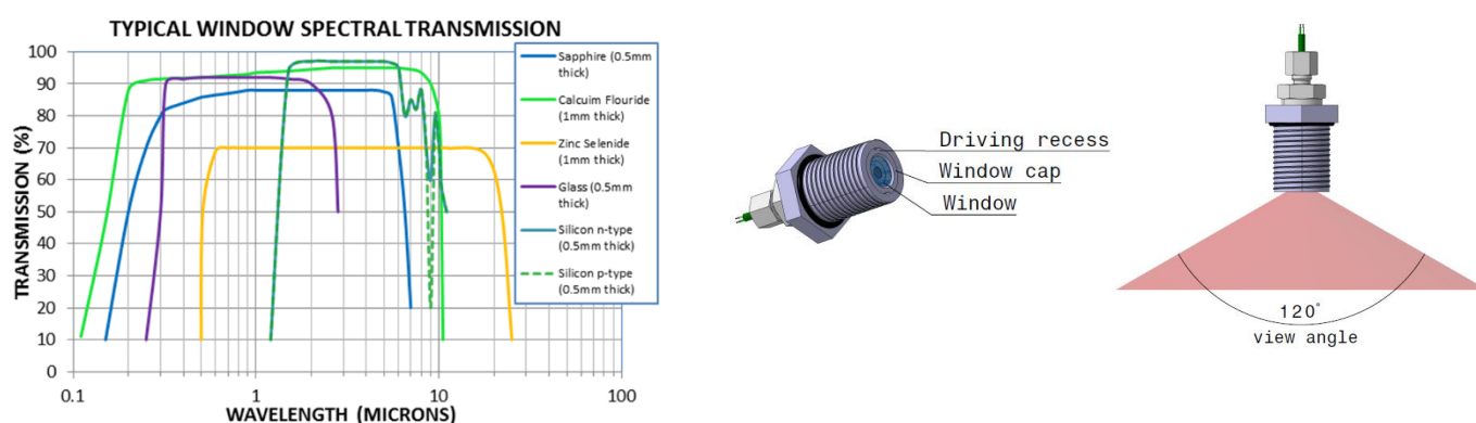
Fig.6 Fluxmètre radiatif : spectre de transmission à prendre en considération et aménagement du capteur
