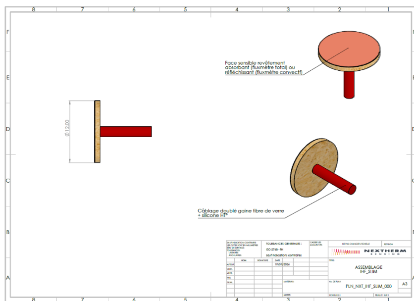
Fig.5 Fluxmètre IHF pastille « SLIM » à pose libre
