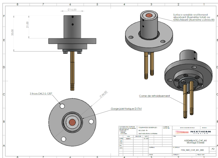
Fig.4 Fluxmètre CHF en interface mécanique à bride 3 trous à 120° (référence M1)
